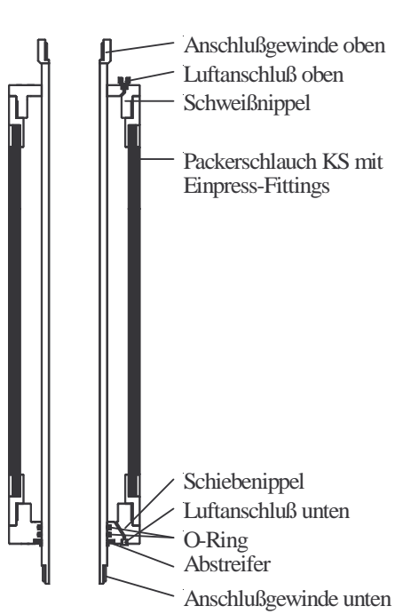
Einfachpacker (Schnitt)
