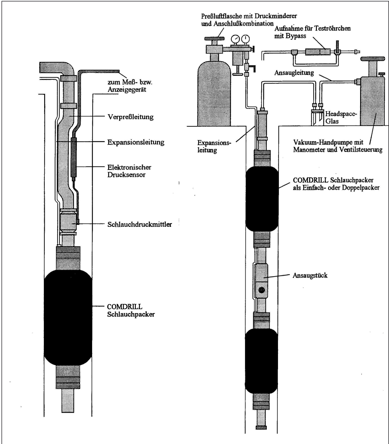
Einfachpacker mit Schlauchdruckmittler
