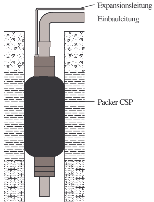
Einfachpacker
